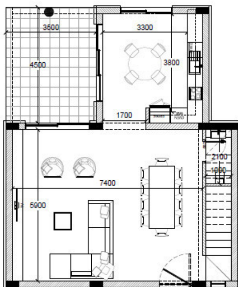
ΚΑΤΟΨΗ ΙΣΟΓΕΙΟΥ
