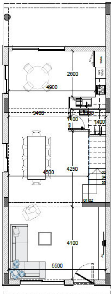
ΚΑΤΟΨΗ ΙΣΟΓΕΙΟΥ
