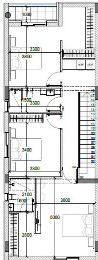
ΚΑΤΟΨΗ ΟΡΟΦΟΥ
