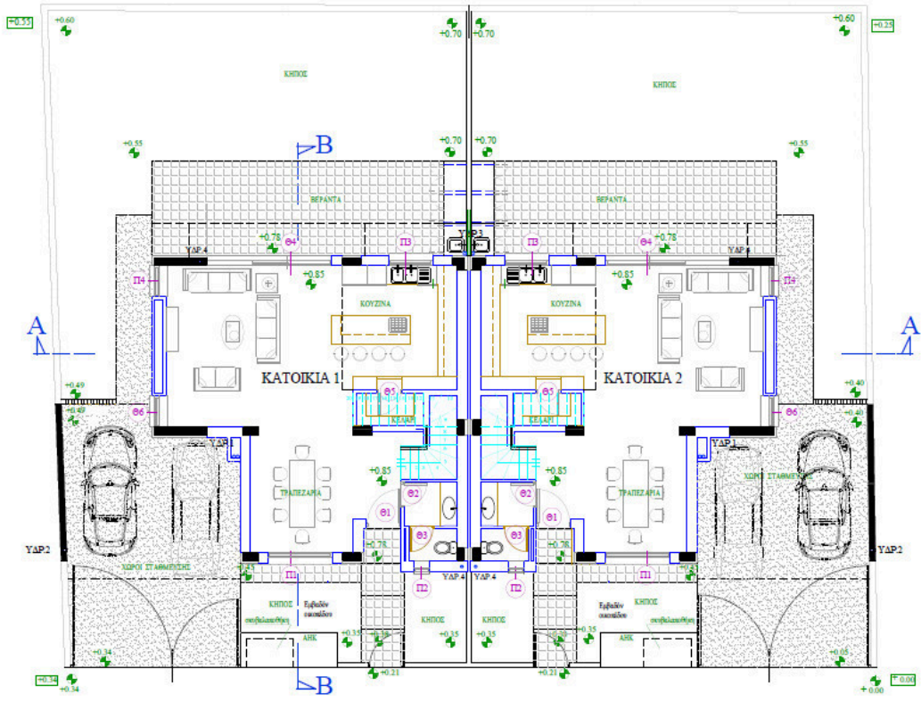
ΚΑΤΟΨΗ ΙΣΟΓΕΙΟΥ ΚΑ. 1:100
