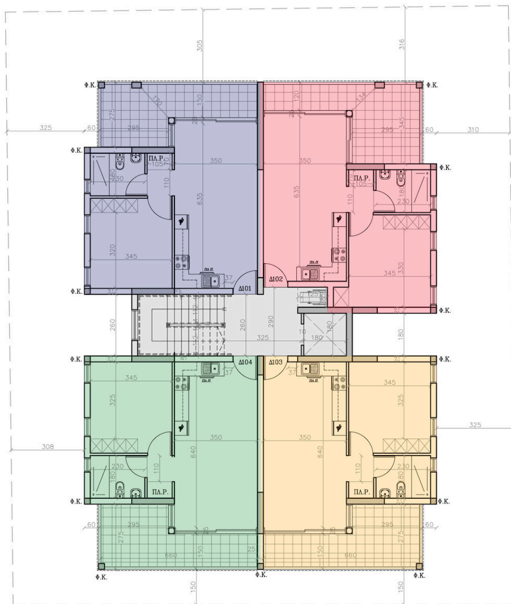
ΚΑΤΟΨΗ 2ΟΥ ΟΡΟΦΟΥ scale 1:100
