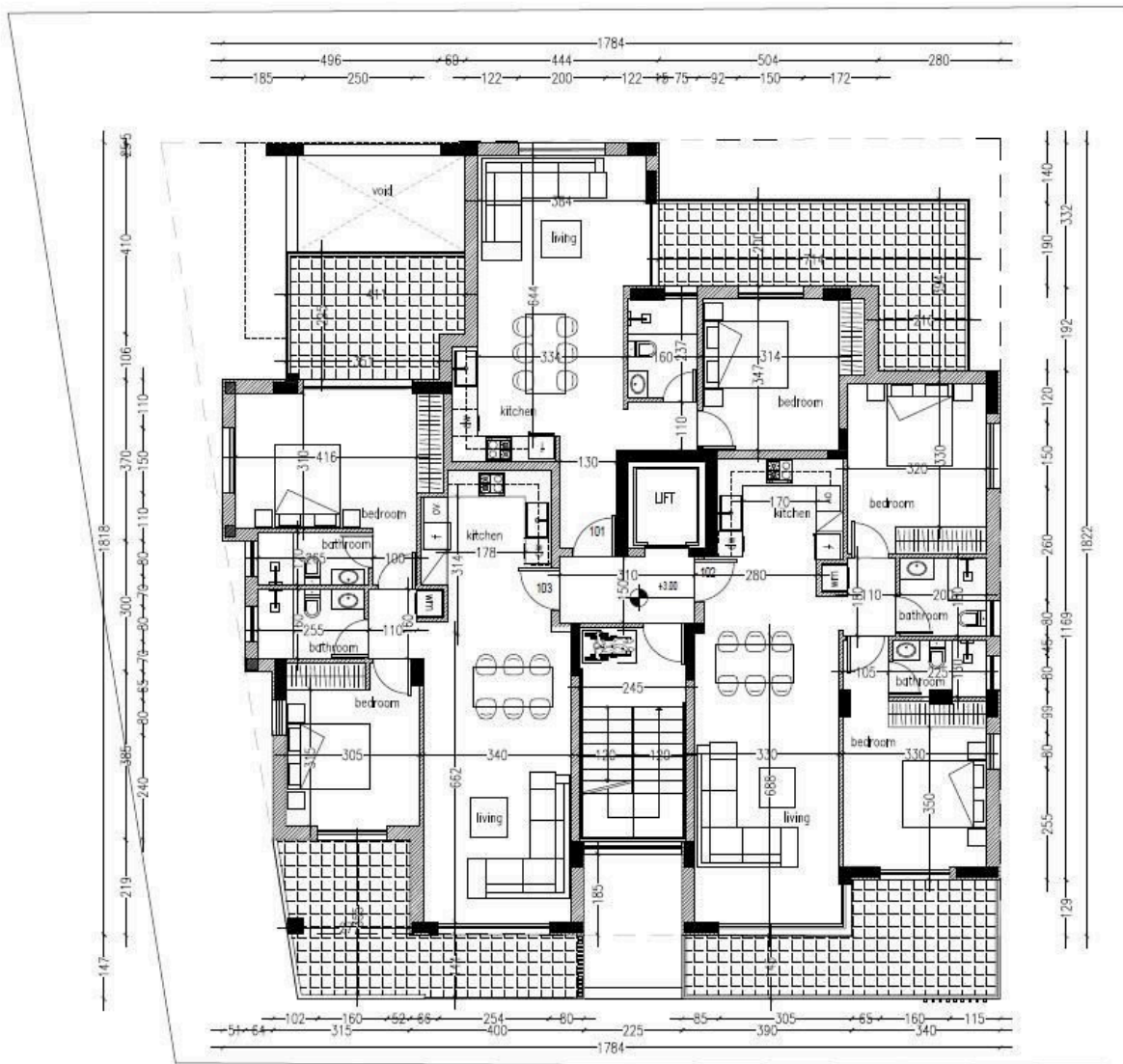
ΚΑΤΟΨΗ 1ΟΥ ΟΡΟΦΟΥ Ι
