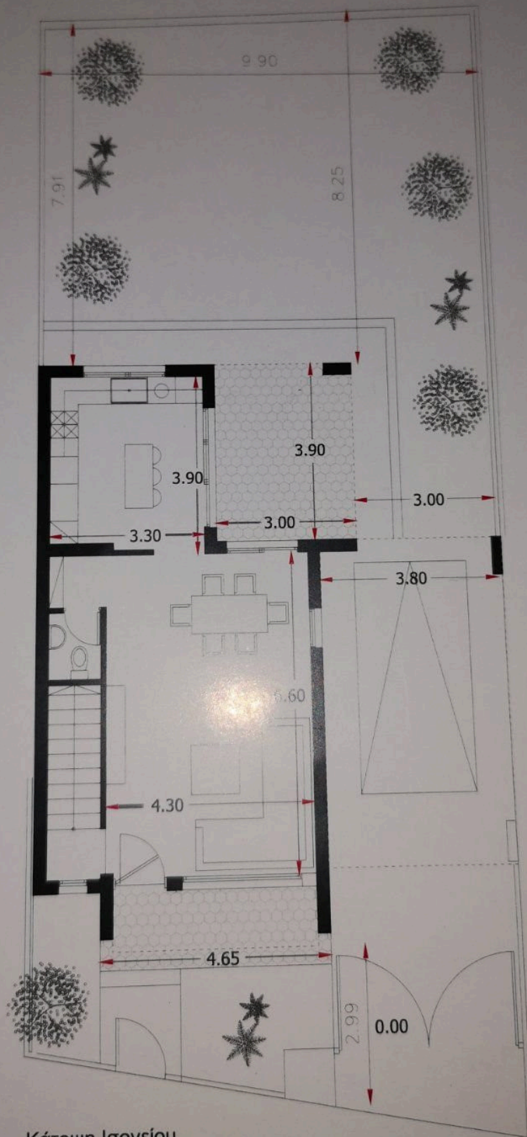
Κάτοψη Ισογείου
