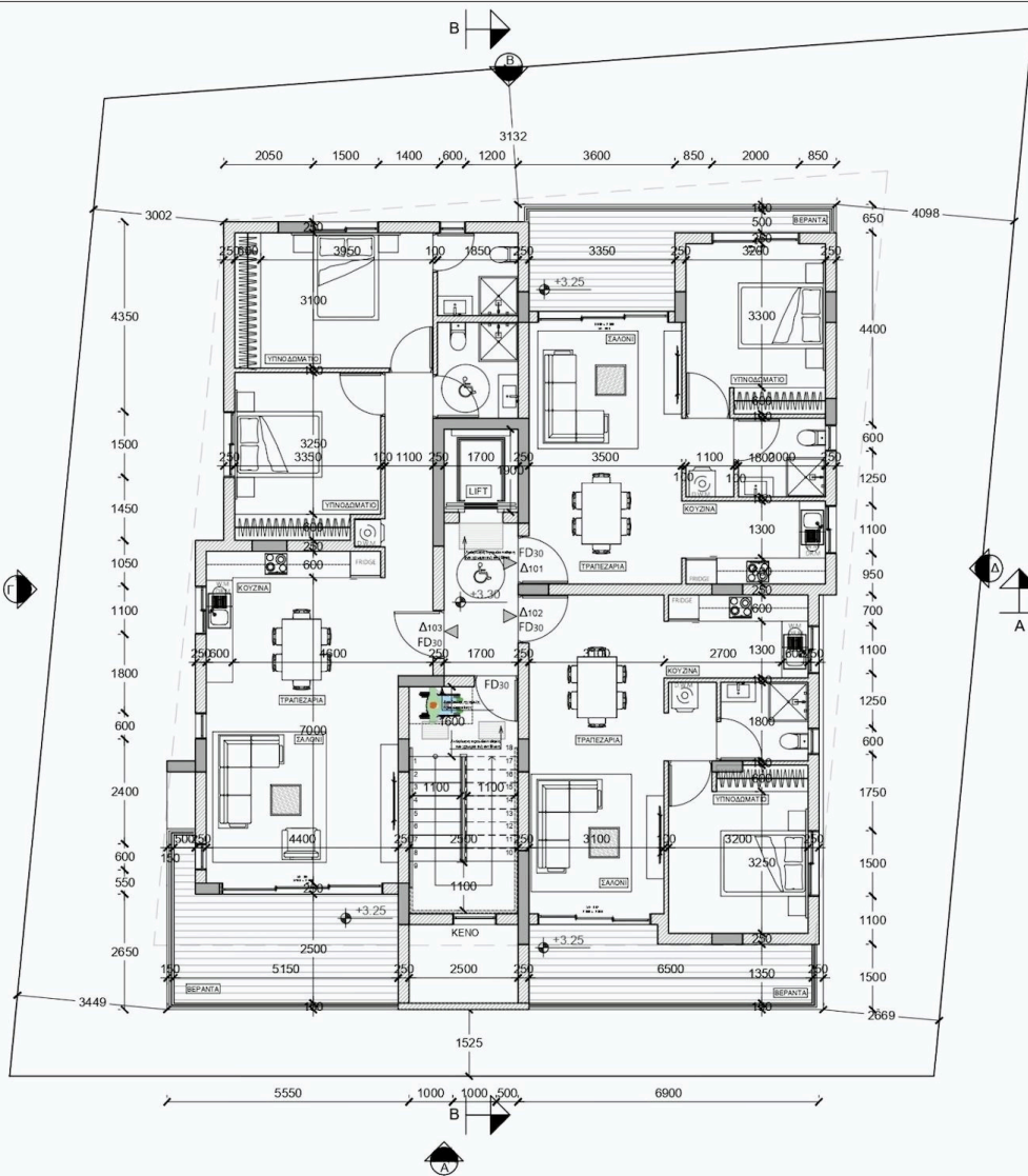
ΚΑΤΩΦΗ 1ΟΥ ΟΡΟΦΟΥ
