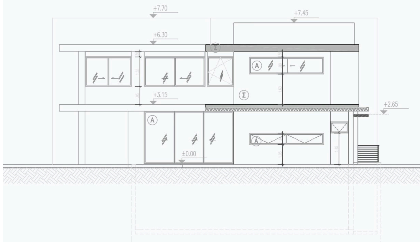
ΝΟΤΙΟΑΝΑΤΟΛΙΚΗ ΟΨΗ - ΠΛΑΓΙΑ ΟΨΗ
