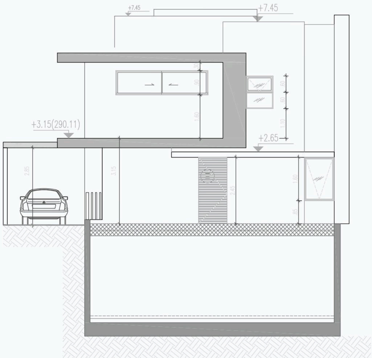
ΒΟΡΕΙΟΑΝΑΤΟΛΙΚΗ ΟΨΗ - ΠΡΟΣΟΨΗ
