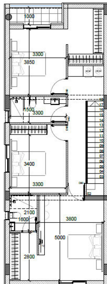
ΚΑΤΟΨΗ ΟΡΟΦΟΥ
