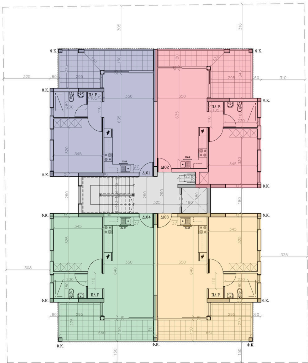
ΚΑΤΩΦΗ 2ΟΥ ΟΡΟΦΟΥ scale 1:100
