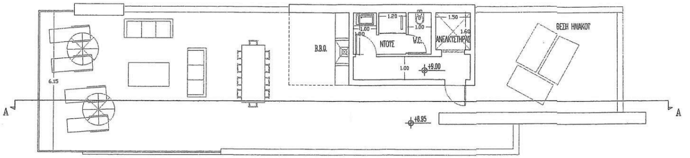
ΚΑΤΟΨΗ ΟΡΟΦΗΣ ΚΑΤΟΙΚΙΑΣ 2
