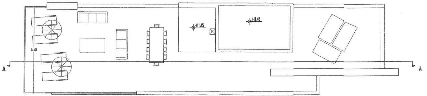
ΚΑΤΟΨΗ ΟΡΟΦΗΣ ΚΛΙΜΑΚΟΣΤΑΣΙΟΥ ΚΑΤΟΙΚΙΑΣ 2
