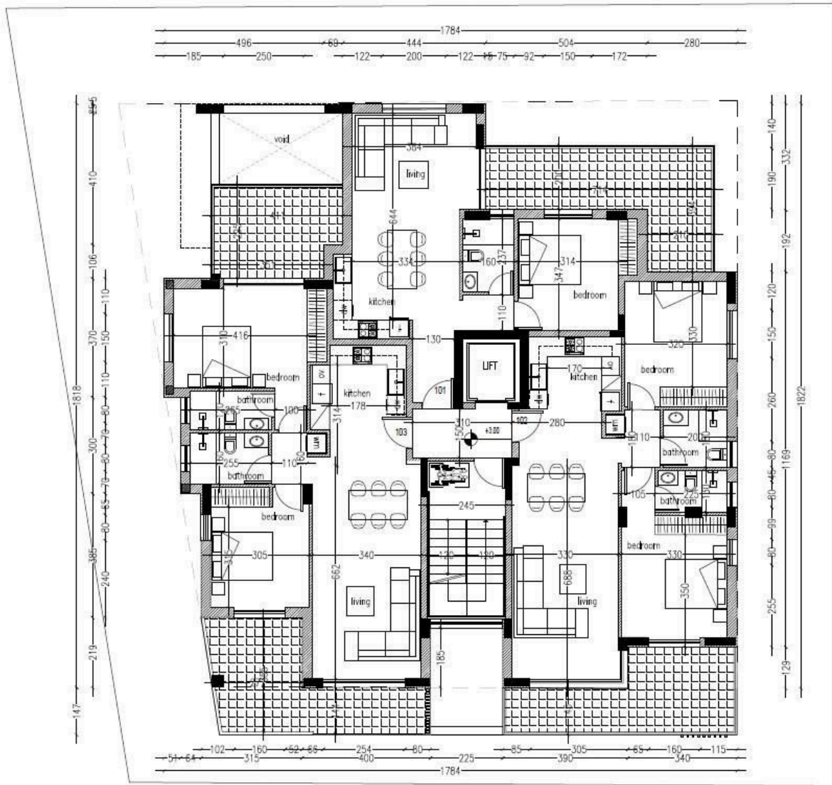
ΚΑΤΟΨΗ 1ΟΥ ΟΡΟΦΟΥ I
