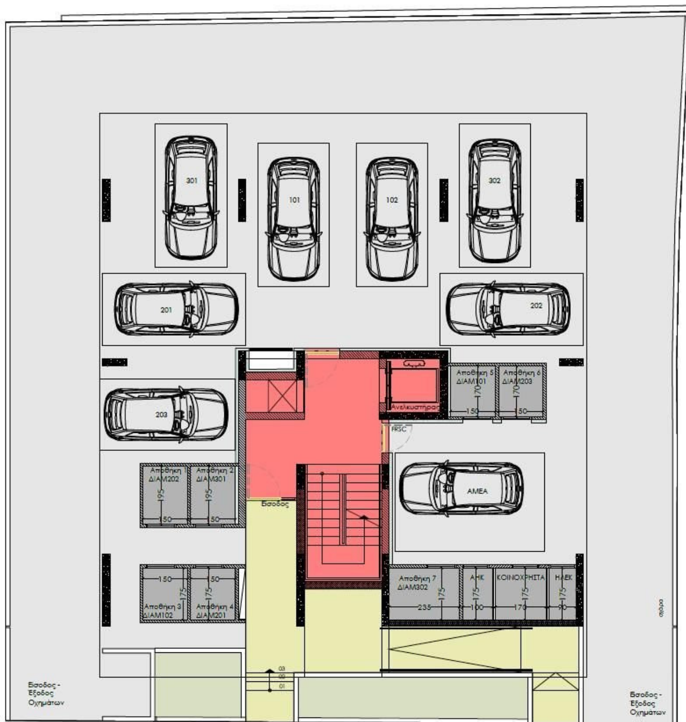
Κάτοψη ισογείου
