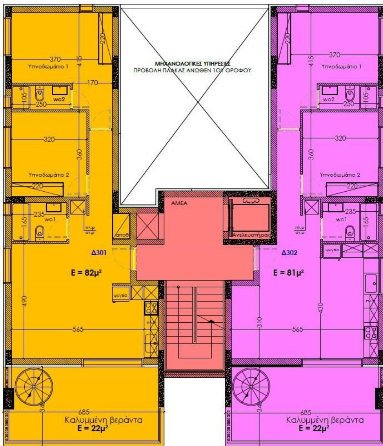
Κάτοψη 3ου ορόφου
