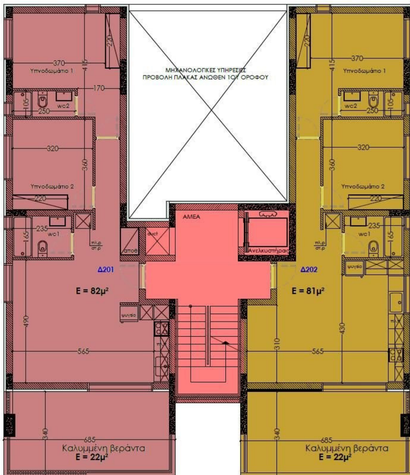
Κάτοψη 2ου ορόφου
