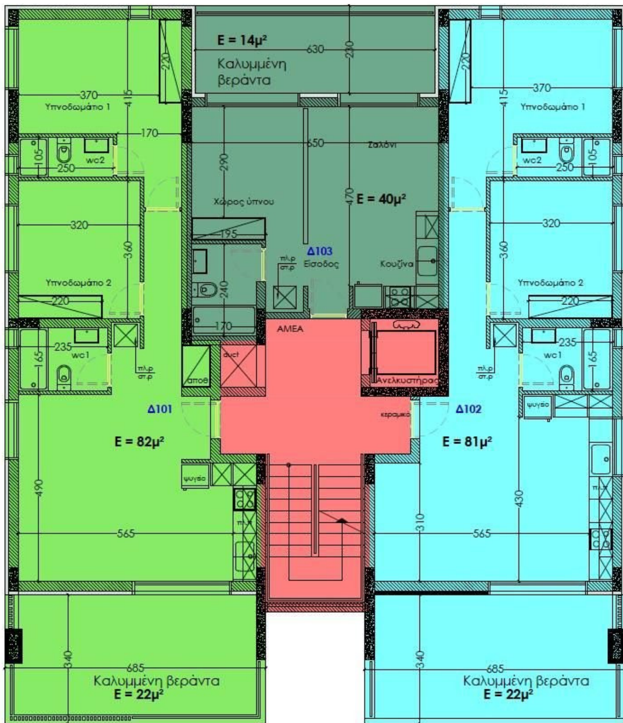
Κάτοψη 1ου ορόφου
