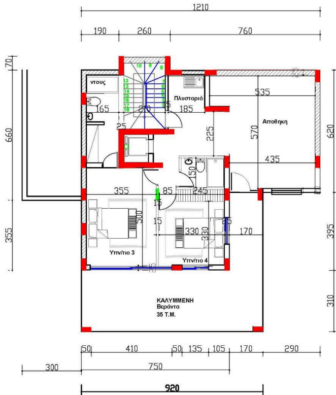
ΚΑΤΟΨΗ ΥΠΟΓΕΙΟΥ ΔΙΑΣΤΑΣΕΙΣ
