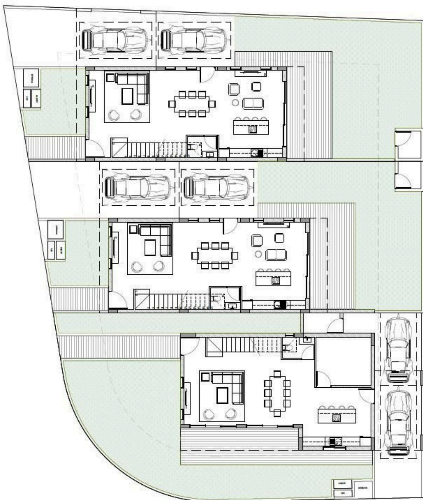
ΟΙΚΟΠΕΔΟ 1 - ΙΣΟΓΕΙΟ
