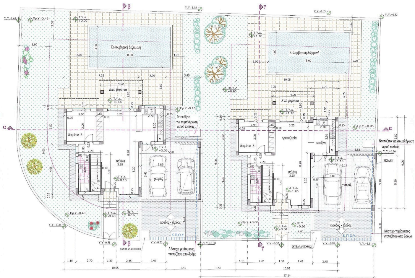
Κάτοψη ισογείου.
