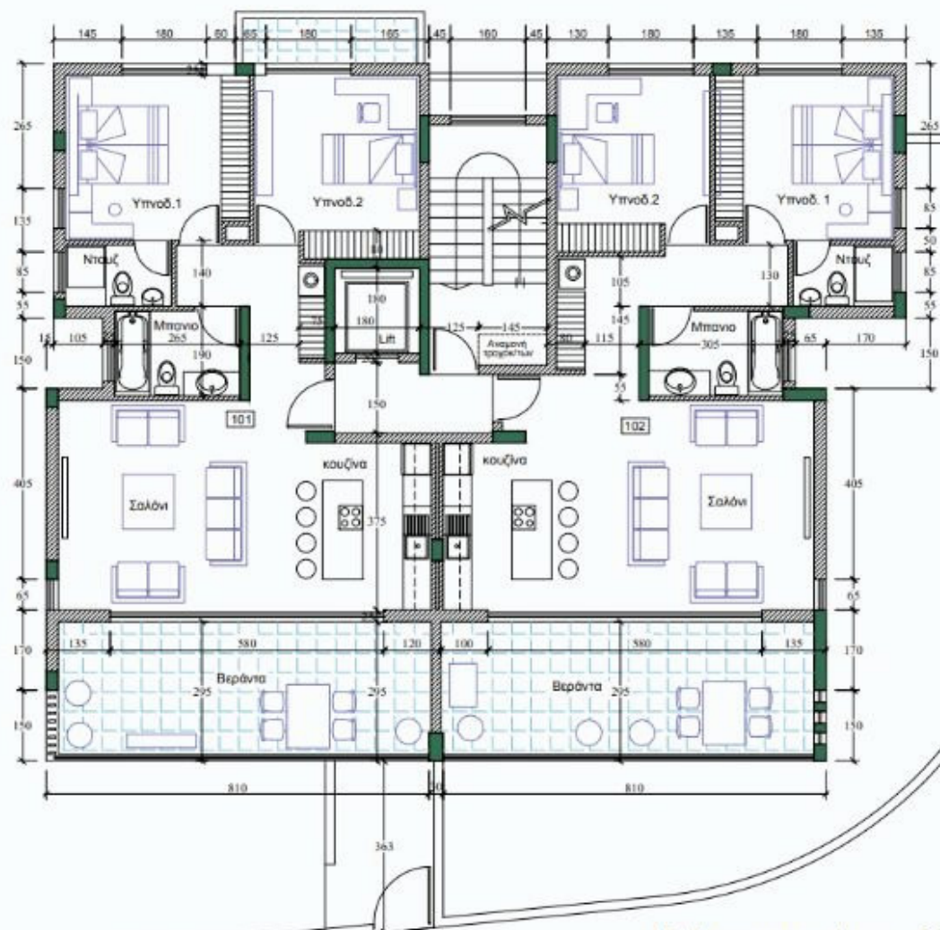
Κάτοψη 1ου Ορόφου
