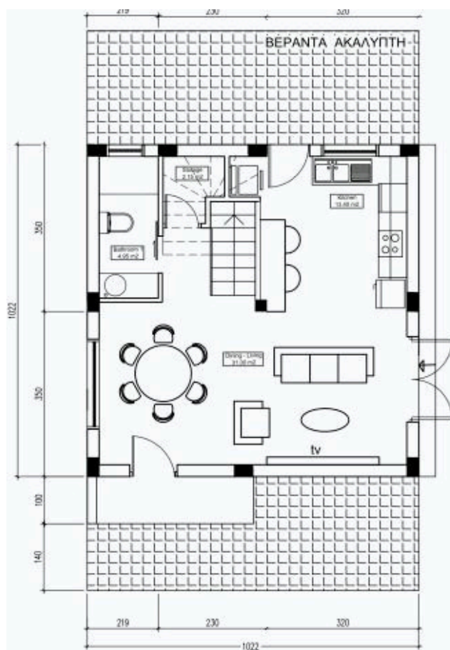
ΚΑΤΟΨΗ ΙΣΟΓΕΙΟΥ
