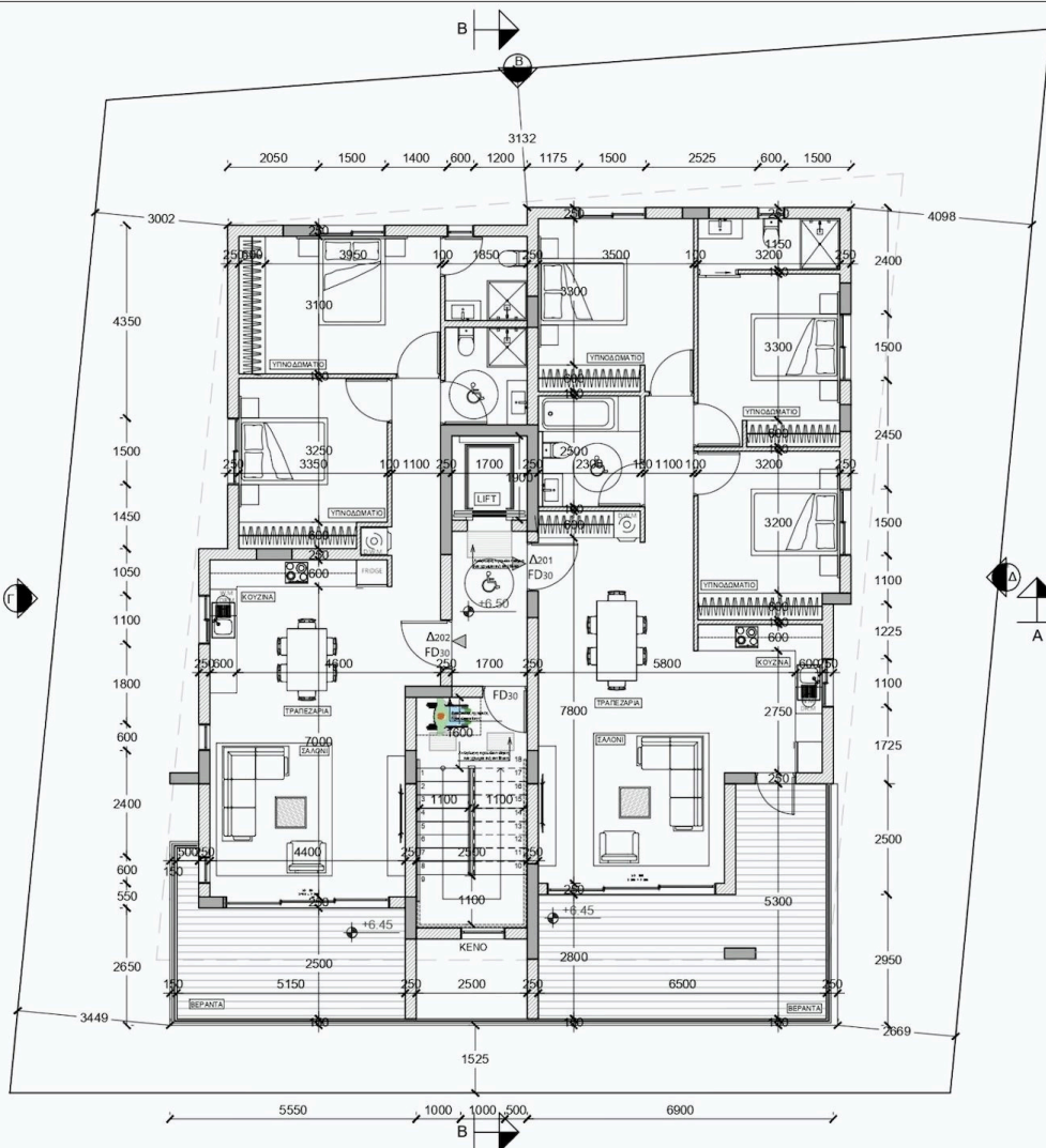
ΚΑΤΟΨΗ 2ΟΥ ΟΡΟΦΟΥ
