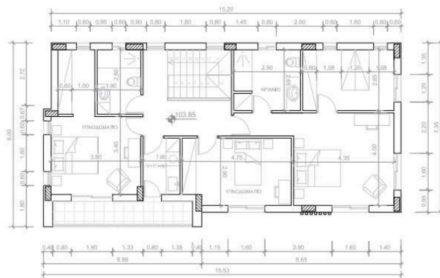
ΚΑΤΟΨΗ ΟΡΟΦΟΥ ΚΑΤΟΙΚΙΑ "Α"
