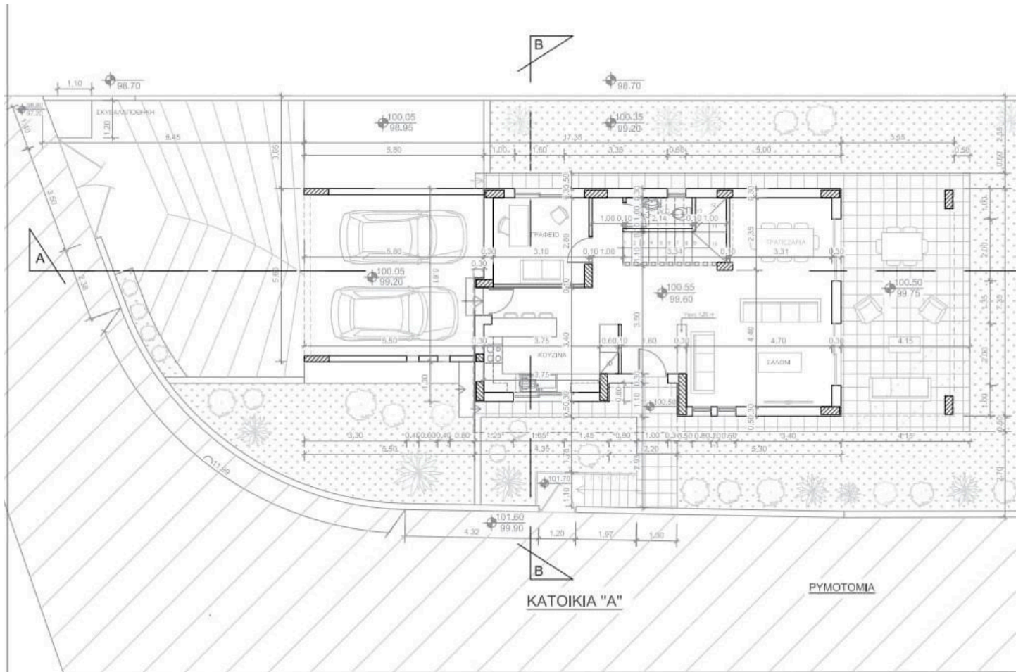
ΚΑΤΟΨΗ ΙΣΟΓΕΙΟΥ
