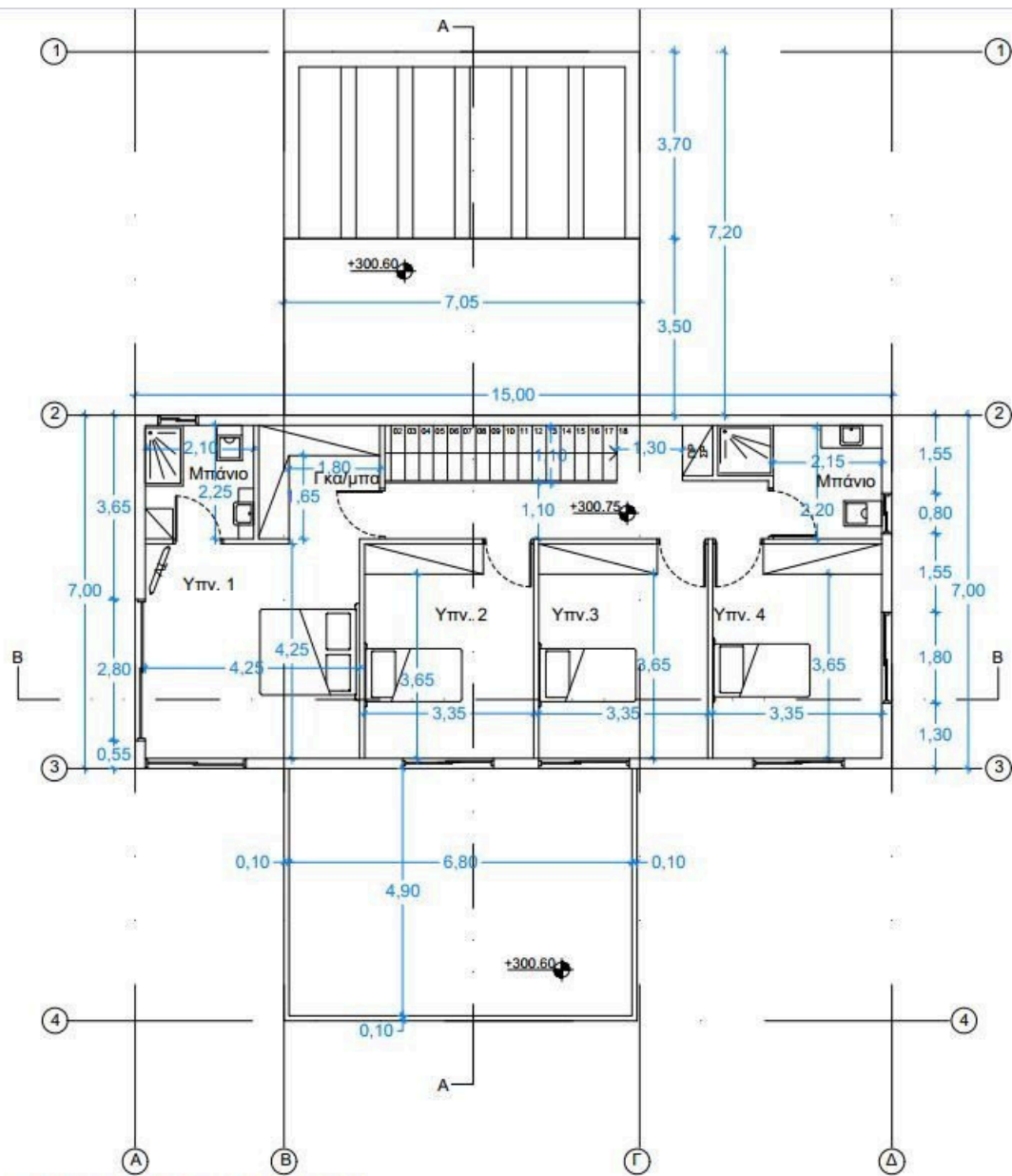
ΚΑΤΟΨΗ ΟΡΟΦΟΥ 1:200
